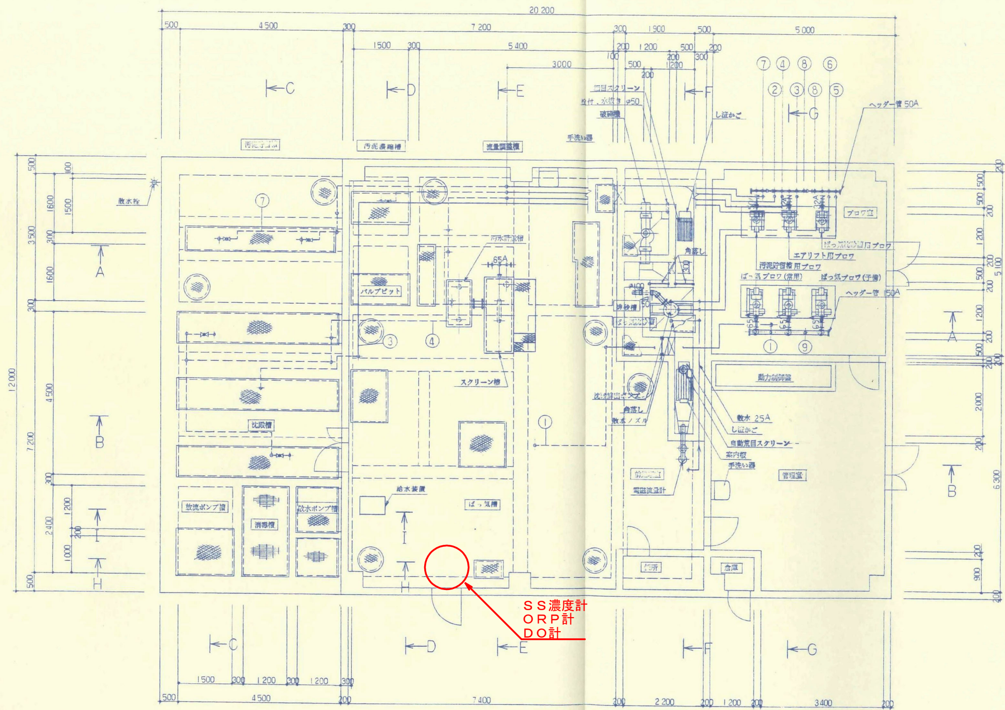
1 階平面図 S = 1/50
