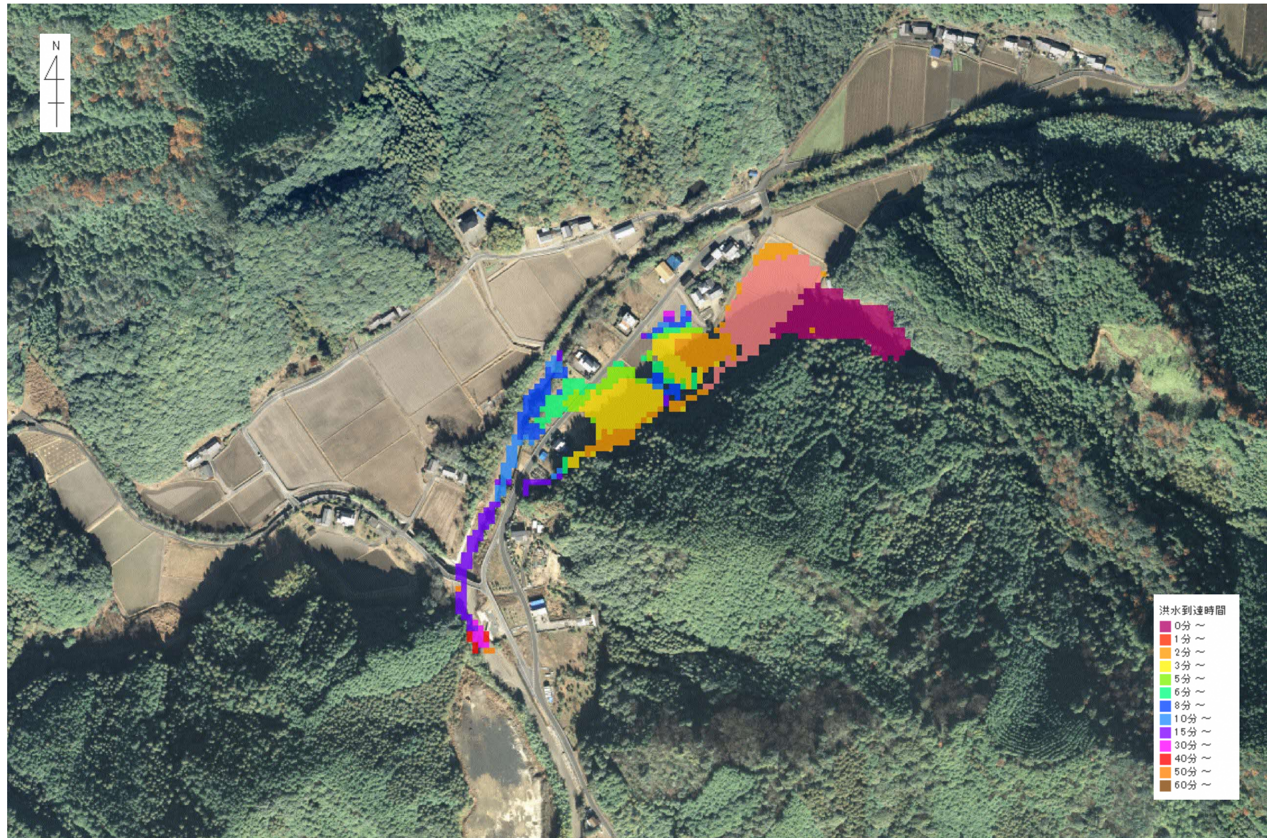
洪水到達時間（樋谷ため池）
