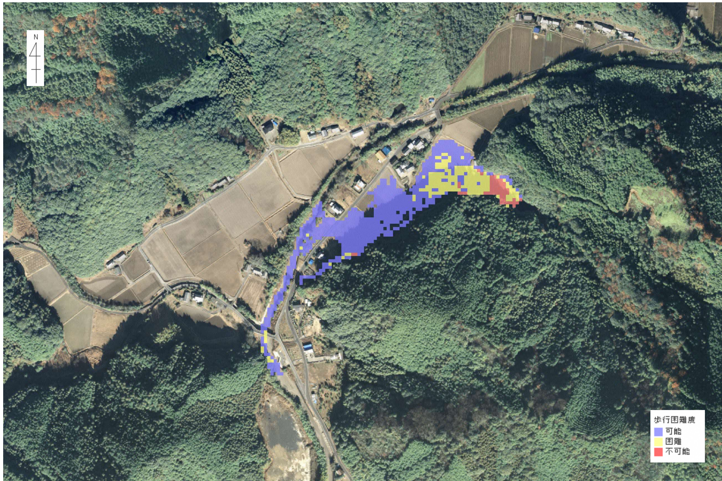
最大歩行困難度 (樋谷ため池)
