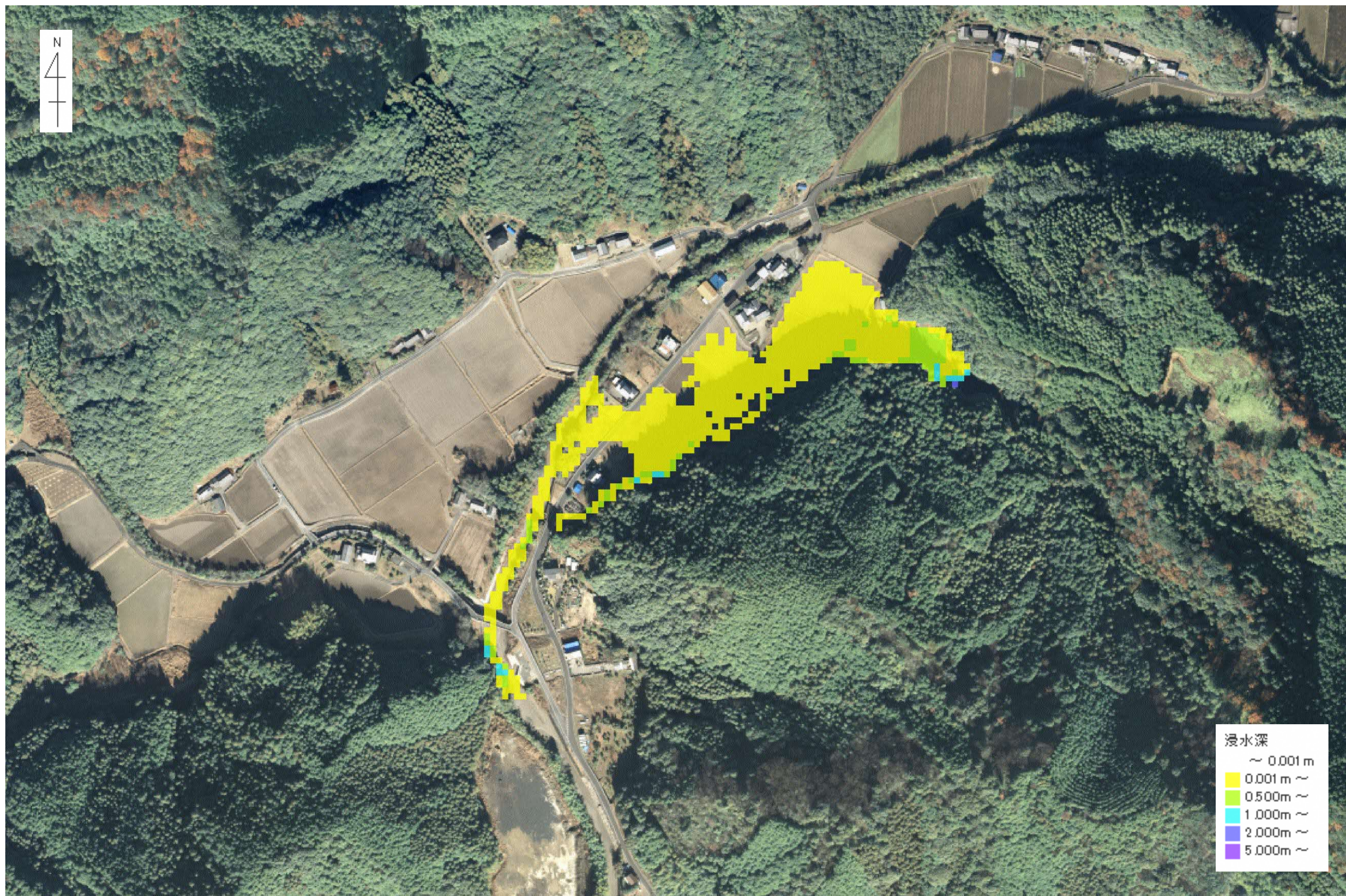
最大浸水深（樋谷ため池）
